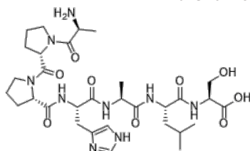
Ala-Pro-Pro-His-Ala-Leu-Ser
